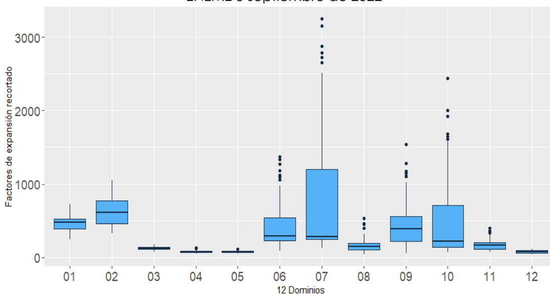
Gráfico 3. Diagramas de caja y bigote del factor de expansión recortados de la ENEMDU septiembre de 2022
