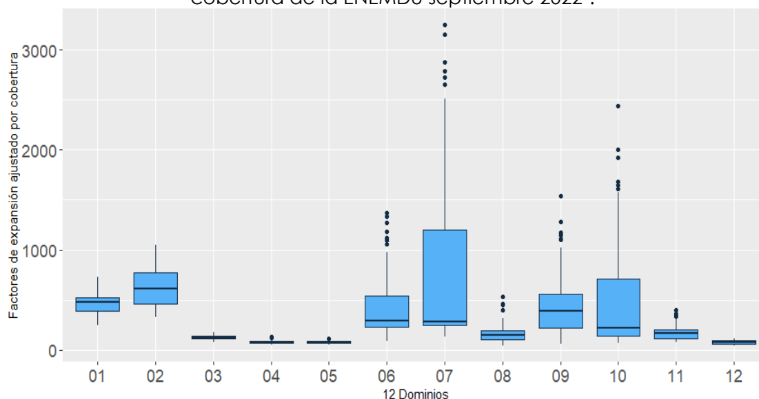
Gráfico 2. Diagramas de caja y bigote de los factores de expansión ajustados por cobertura de la ENEMDU septiembre 2022 1 .
